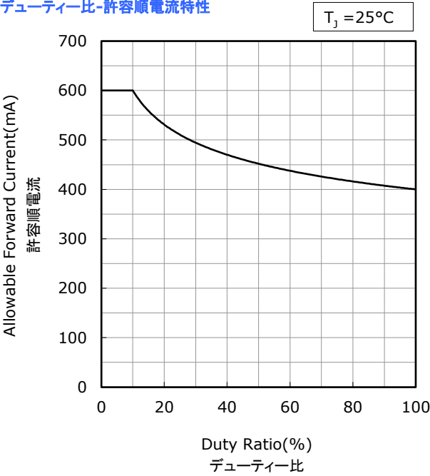
Duty Ratio vs Allowable Forward Current デューティ比-許容順電流特性
